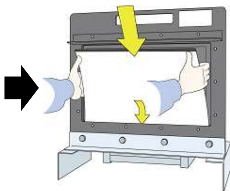
下側のすき間にシートを差込み (イラスト②)
